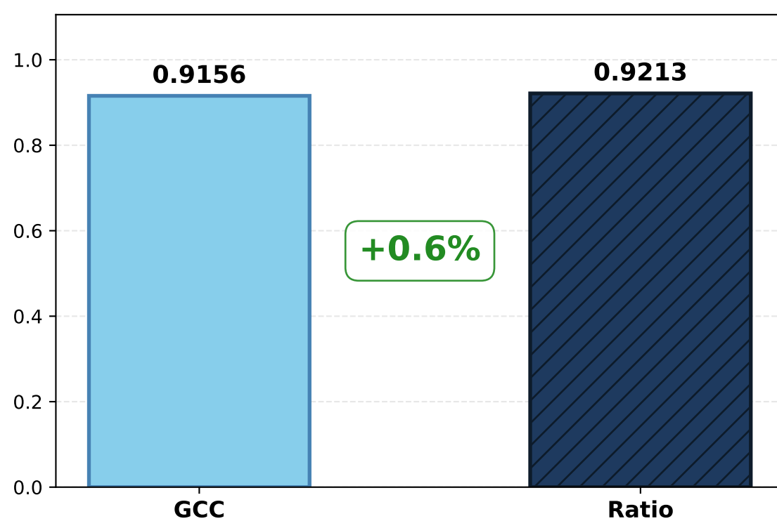
LPIPS
