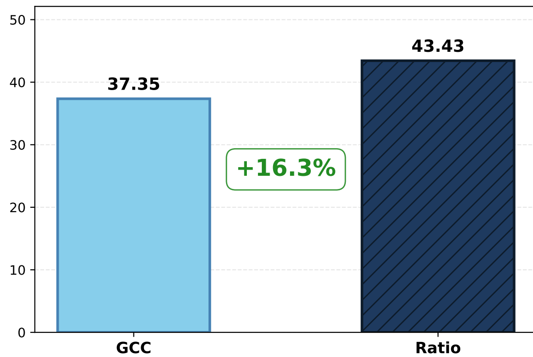
VMAF
