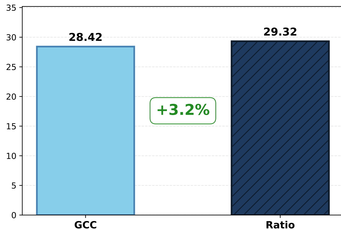
VMAF
