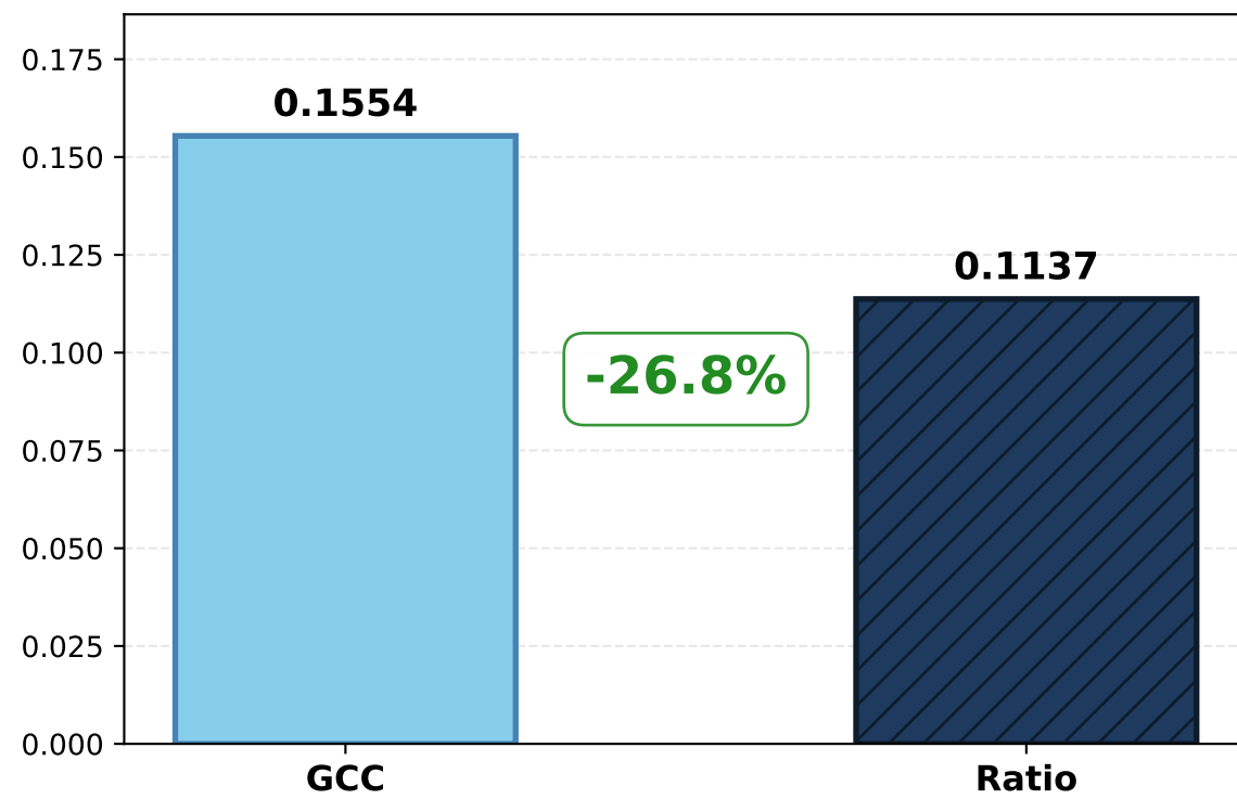
LPIPS
